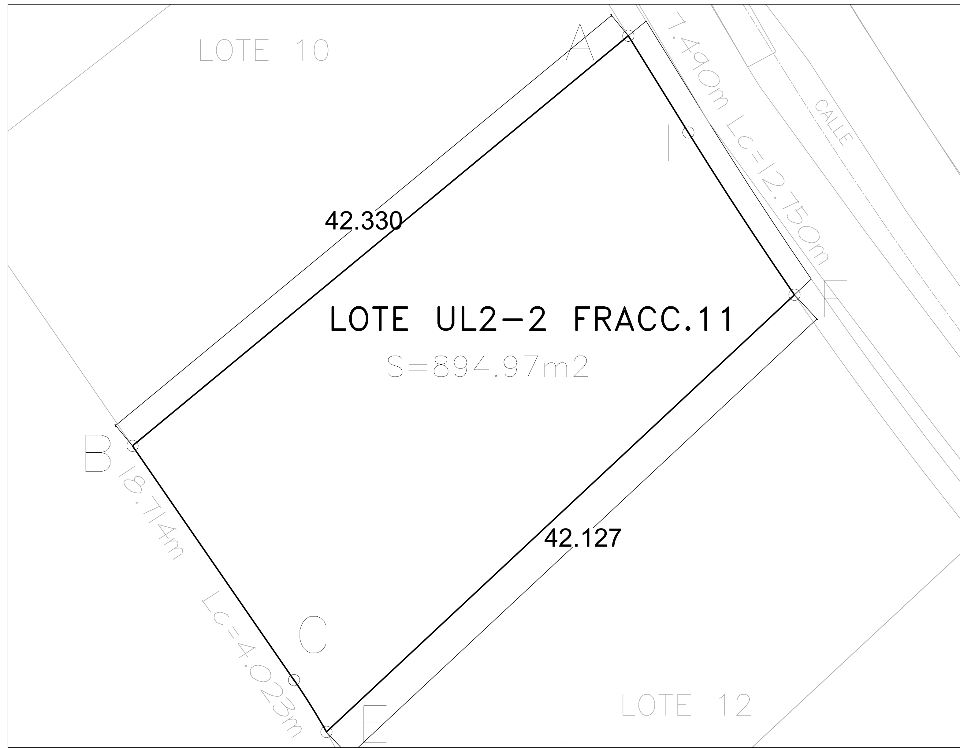
PLANO TOPOGRAFICO ESCALA 1:50
