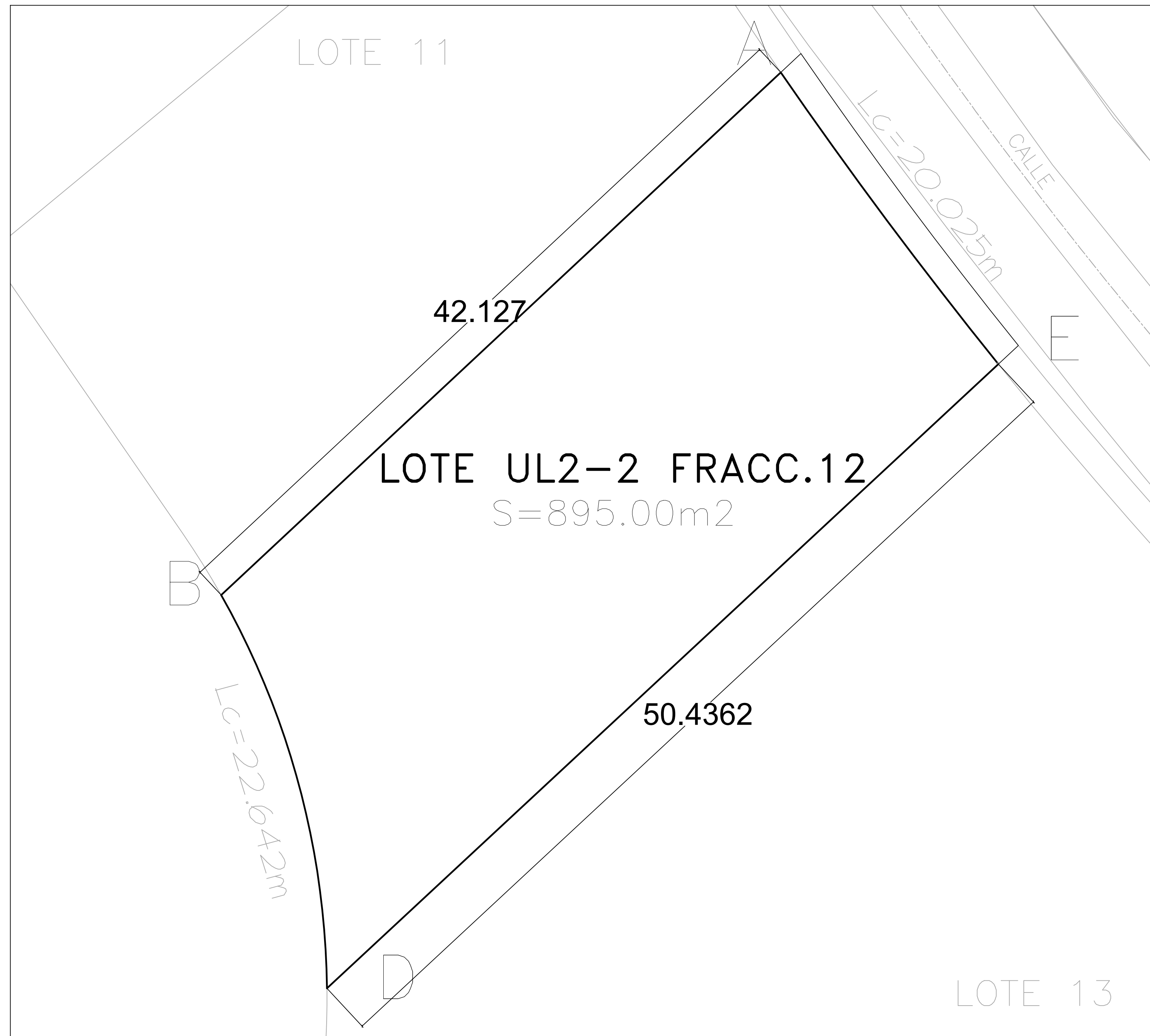
PLANO TOPOGRAFICO ESCALA 1:50
