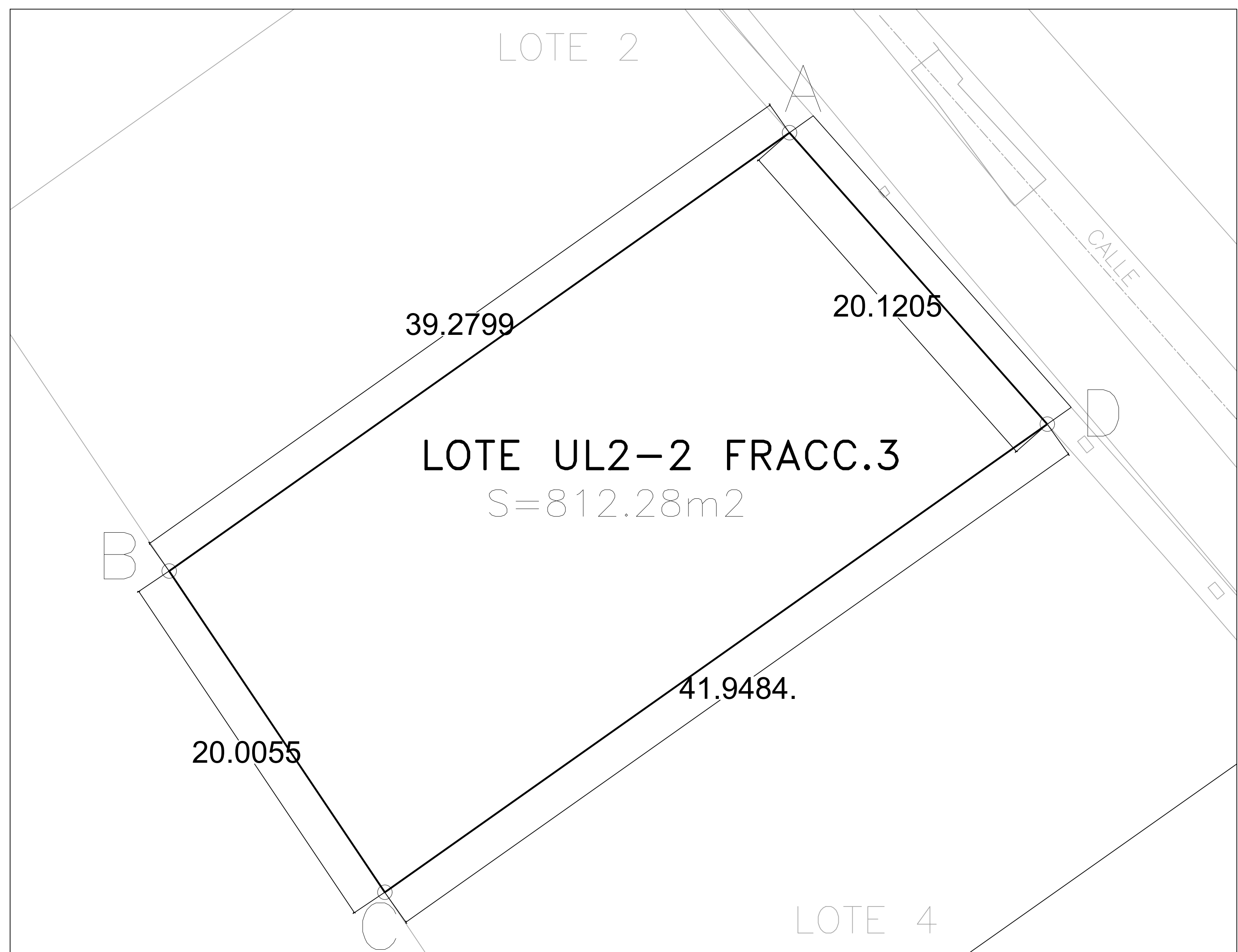
PLANO TOPOGRAFICO ESCALA 1:50
